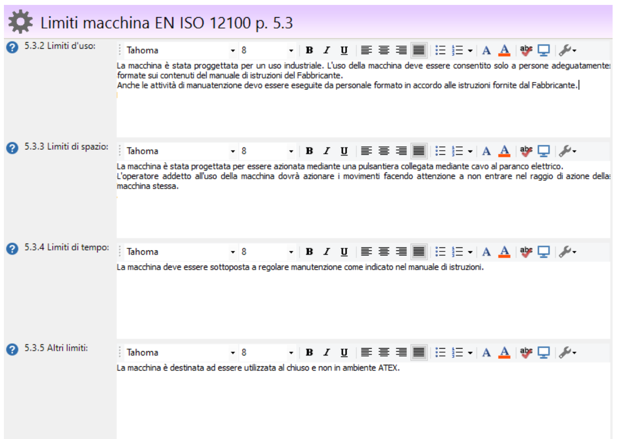
Limiti macchina
