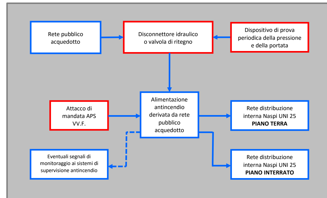
TAV. SCH. 03
