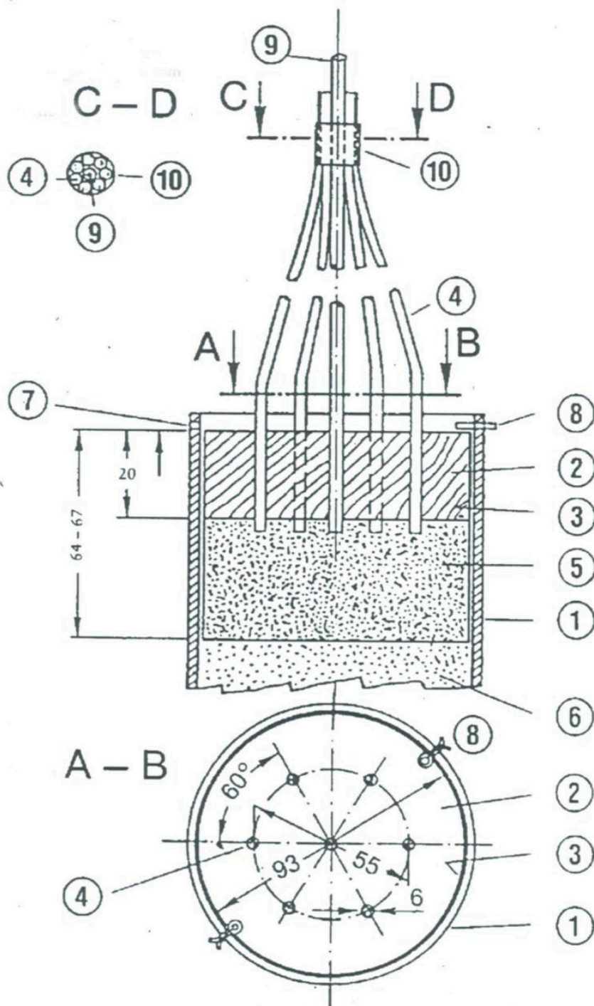
Carica d'innesco con accensione in sette punti
