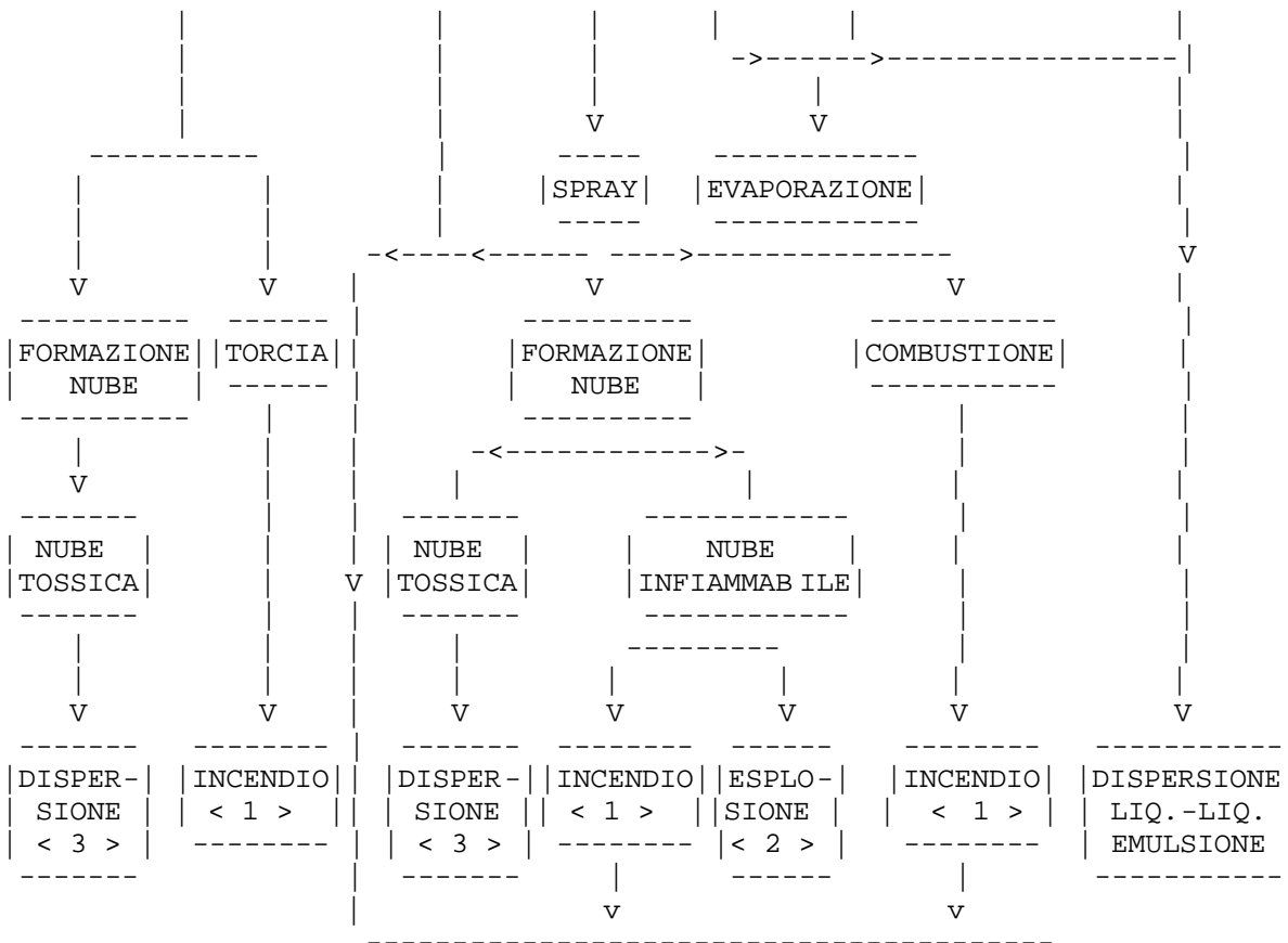
FIGURA 3 - Schema dei rilasci di fluidi
