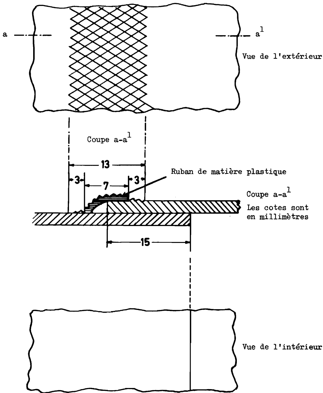
Croquis n° 3 BACHE FAITE DE PLUSIEURS PIECES ASSEMBLEES PAR SOUDURE
