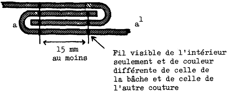
Coupe a-a¹ Couture à double repli
