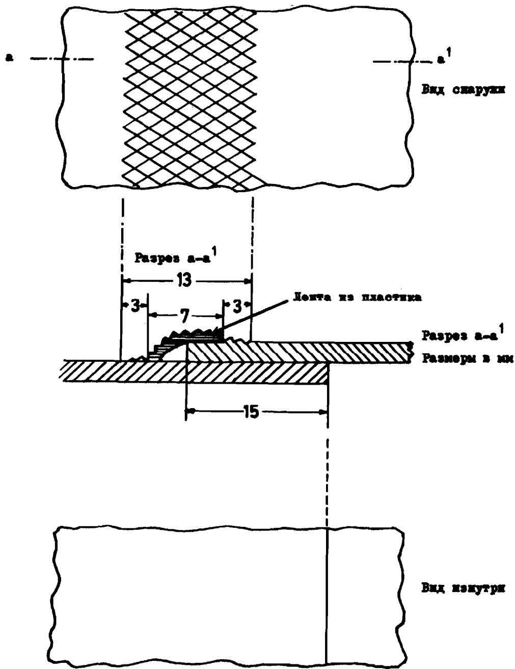
Рис. № 9 БРЕЗЕНТ, ИЗГОТОВЛЕННЫЙ ИЗ НЕСКОЛЬКИХ КУСКОВ ТКАНИ, СОЕДИНЕННЫХ ПОСРЕДСТВОМ СПАЙКИ
