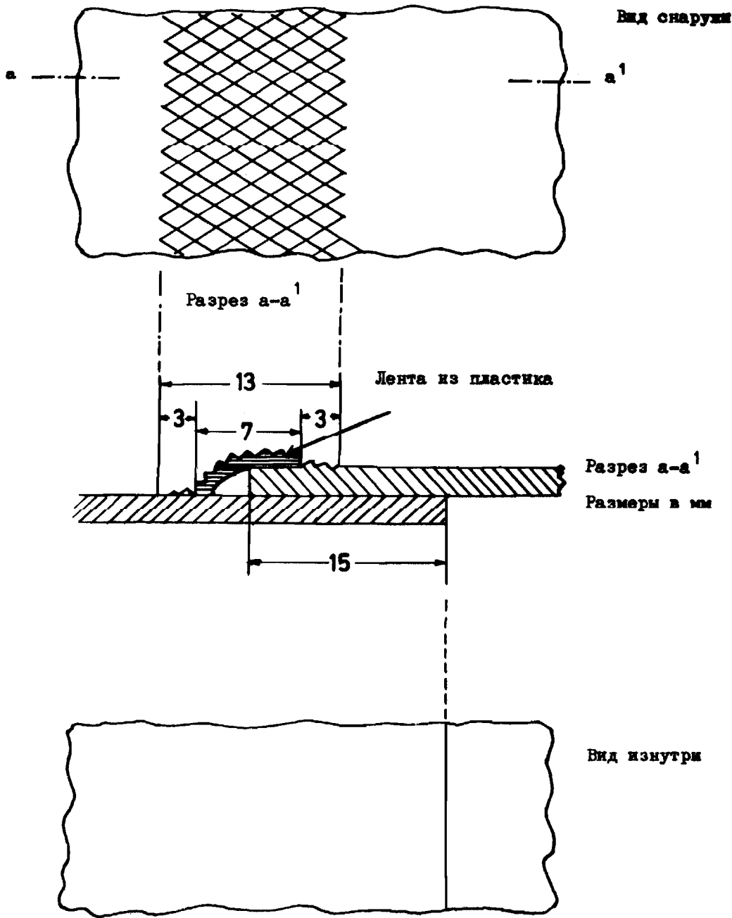
Часть I – Рис. № 3 БРЕЗЕНТ, ИЗГОТОВЛЕННЫЙ ИЗ НЕСКОЛЬКИХ КУСКОВ ТКАНИ, СОЕДИНЕННЫХ ПОСРЕДСТВОМ СПАЙКИ
