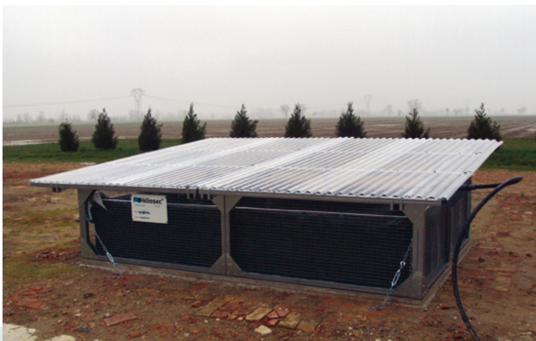
Sistema per la gestione dei reflui di prodotti fitosanitari. (Heliotec®)
