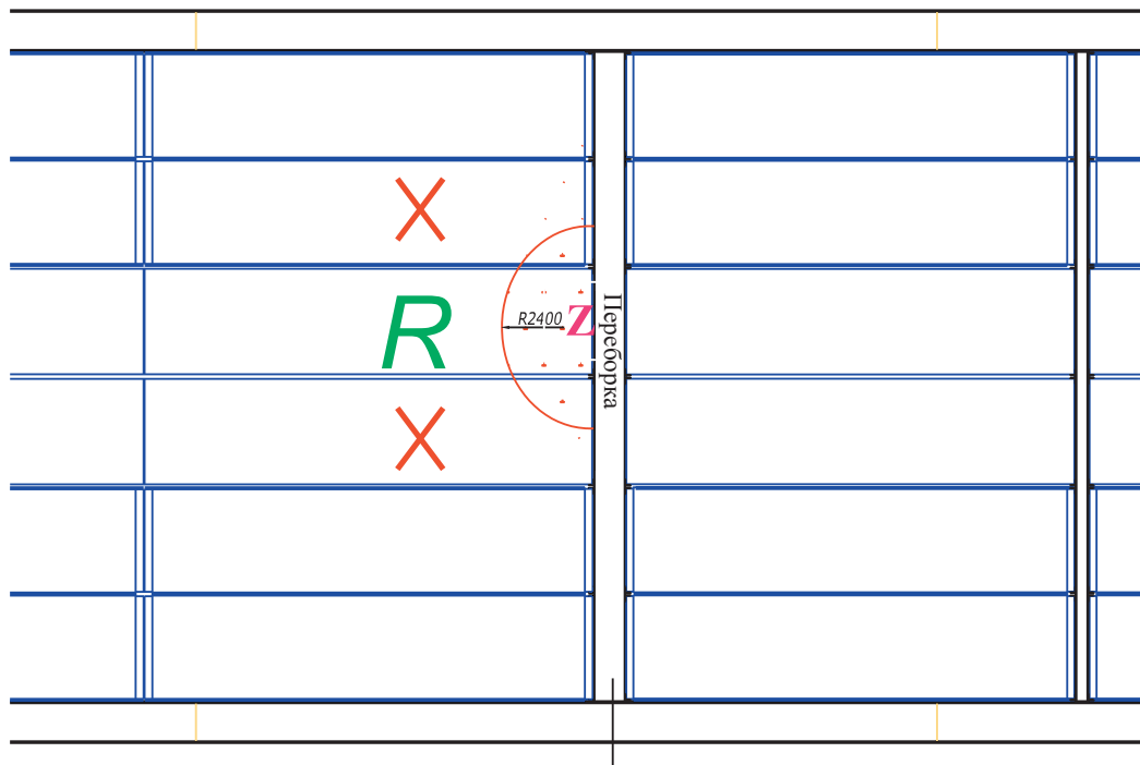
Вид сверху 2. В трюме
