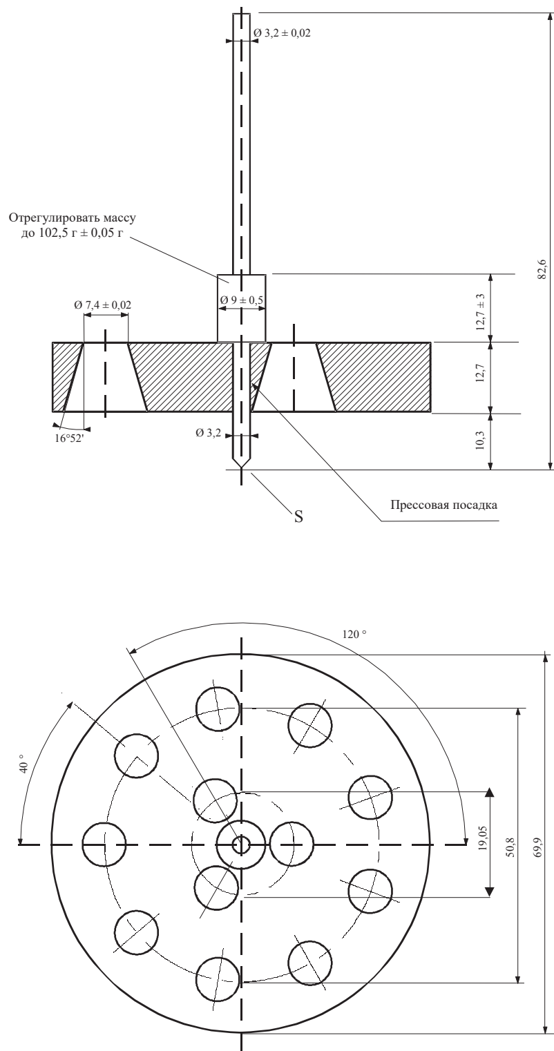
Рис. 1. Пенетрометр
