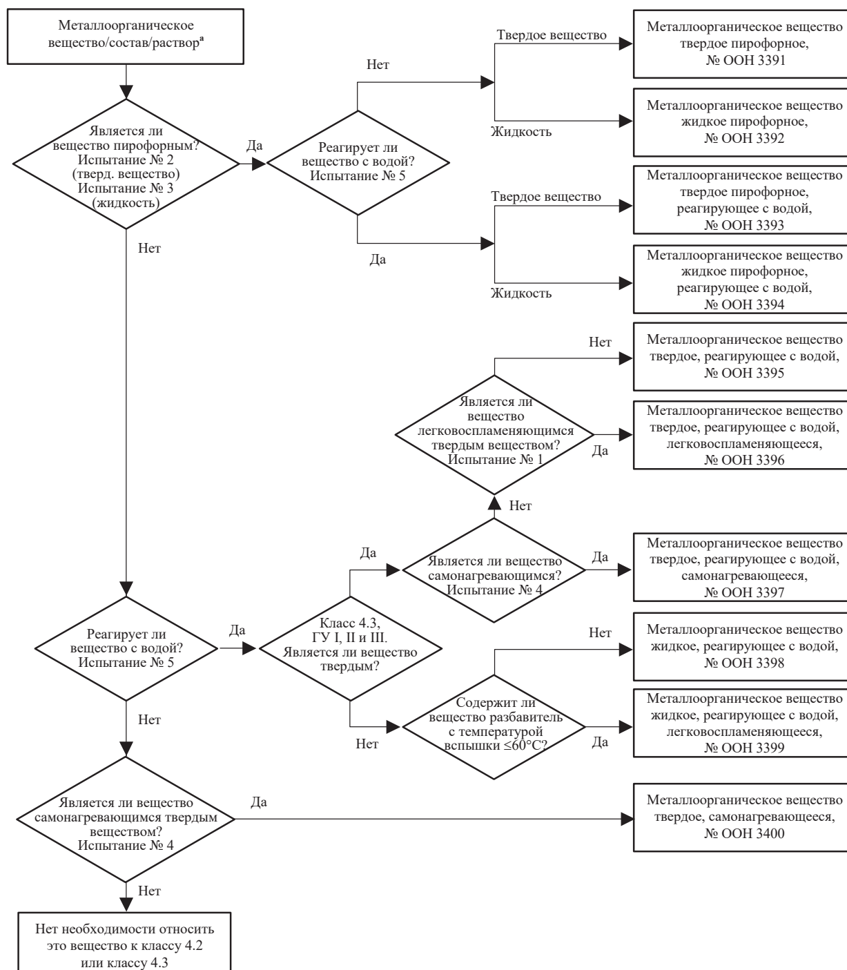
Рис. 2.3.5 Схема принятия решения об отнесении металлоорганических веществ к классам 4.2 и 4.3 b
