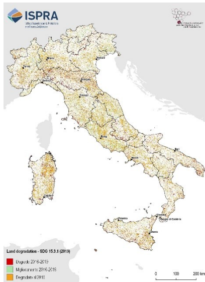
Fig. 14 – Aree degradate durante i periodi di baseline (2000-2015) e periodo di reporting (2016-2019) secondo la metodologia di calcolo SDG 15.3.1
