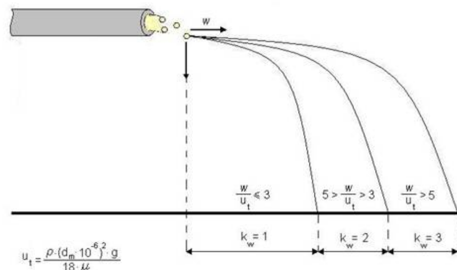
Grafico 3 – Valori del coefficiente k_w in funzione della velocità dell'aria di ventilazione e della velocità di sedimentazione
