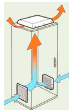
Ventilazione con estrazione aria dal tetto
