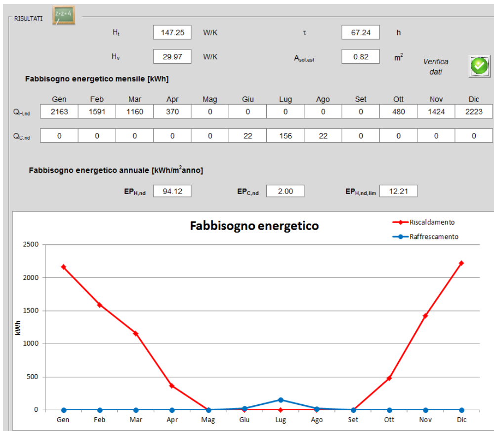
Figura 11. Involucro: Riquadro 8 "Riepilogo Risultati Fabbisogno energia netta"
