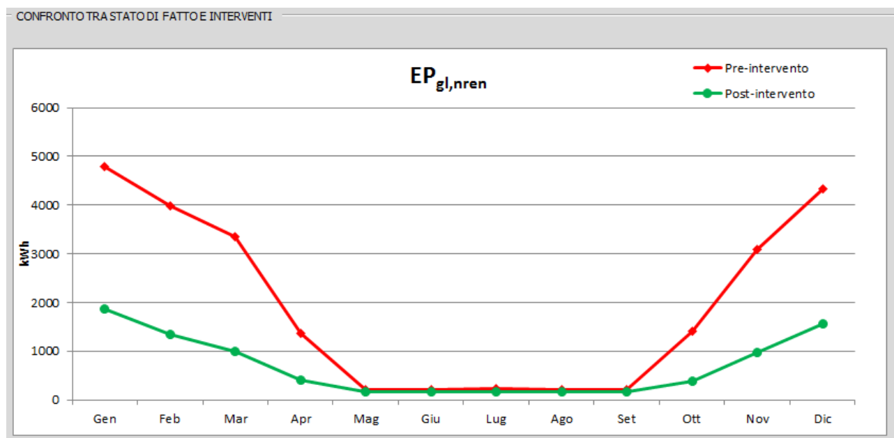
Figura 27. Modulo Raccomandazioni: Confronto prestazioni pre e post interventi di riqualificazione
