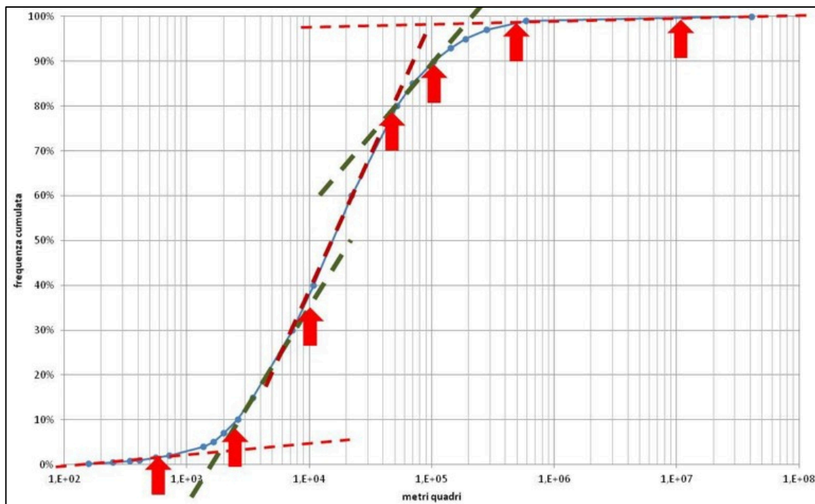
Figura 4-1 - Curva di frequenza cumulata delle superfici delle aree in frana censite nel Progetto IFFI
