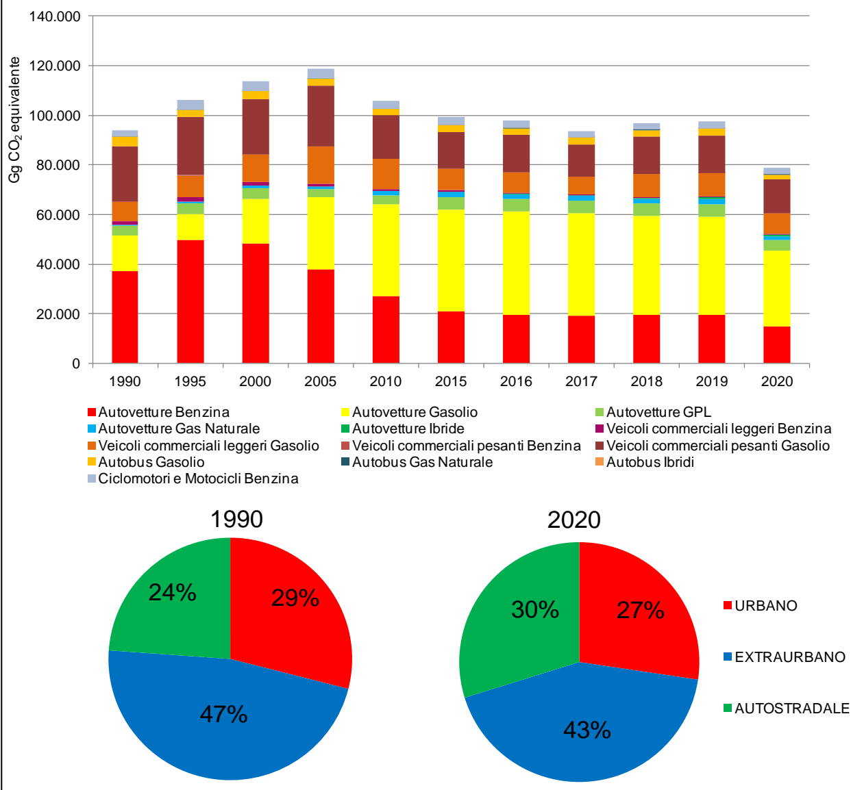
Figura 3: Emissioni di gas serra su strada in Italia dal 1990 al 2020 per tipo di veicolo e ambito di percorrenza (ISPRA 2022)
