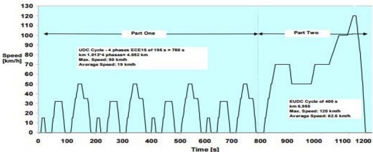
Figura 1: Ciclo NEDC
