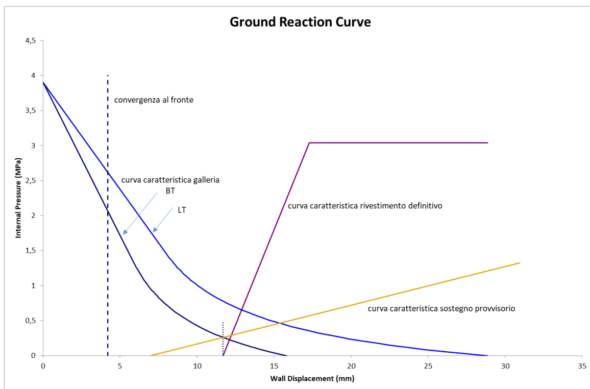
Figura 5.4 – Esempio di applicazione del metodo convergenza-confinamento
