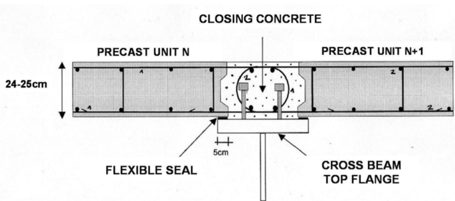
Figura 4.98 – Soluzione di getto con piattabanda della trave che funge da cassero
