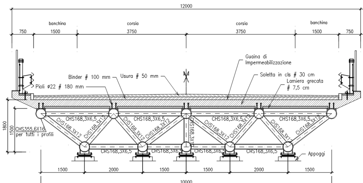
Figura 4.66 - Sezione Tipo
