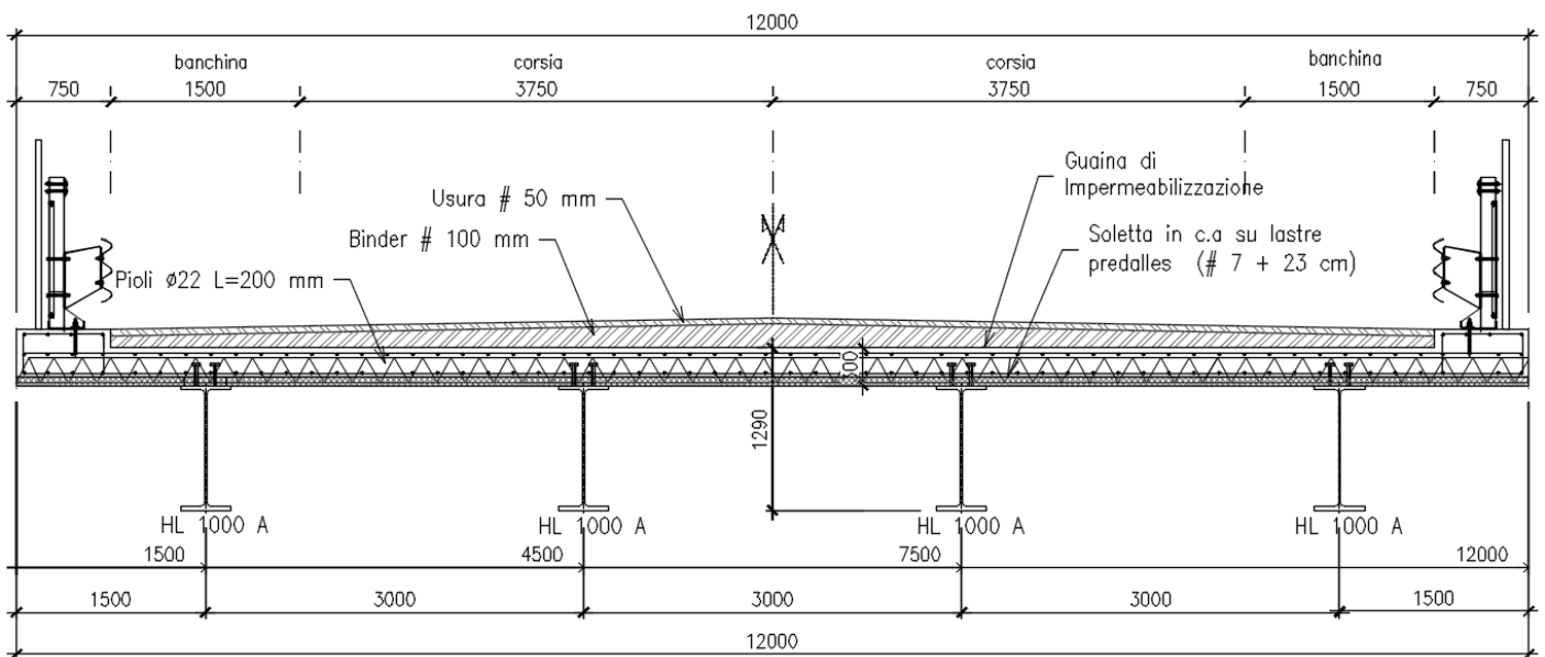
Figura 4.15 - Sezione tipo
