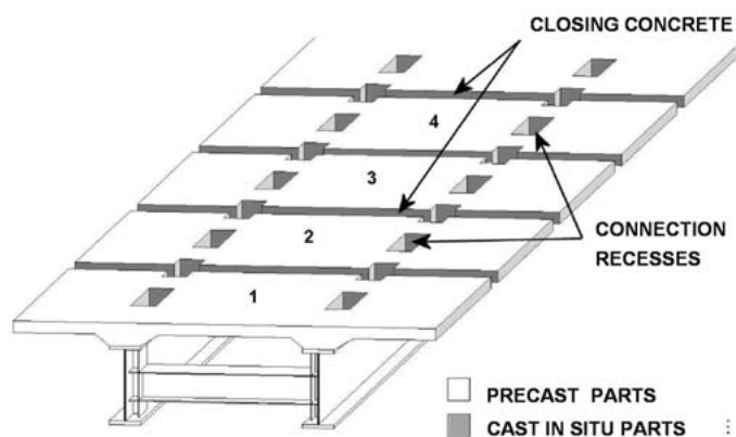
Figura 4.96 - Lastre prefabbricate a tutta larghezza
