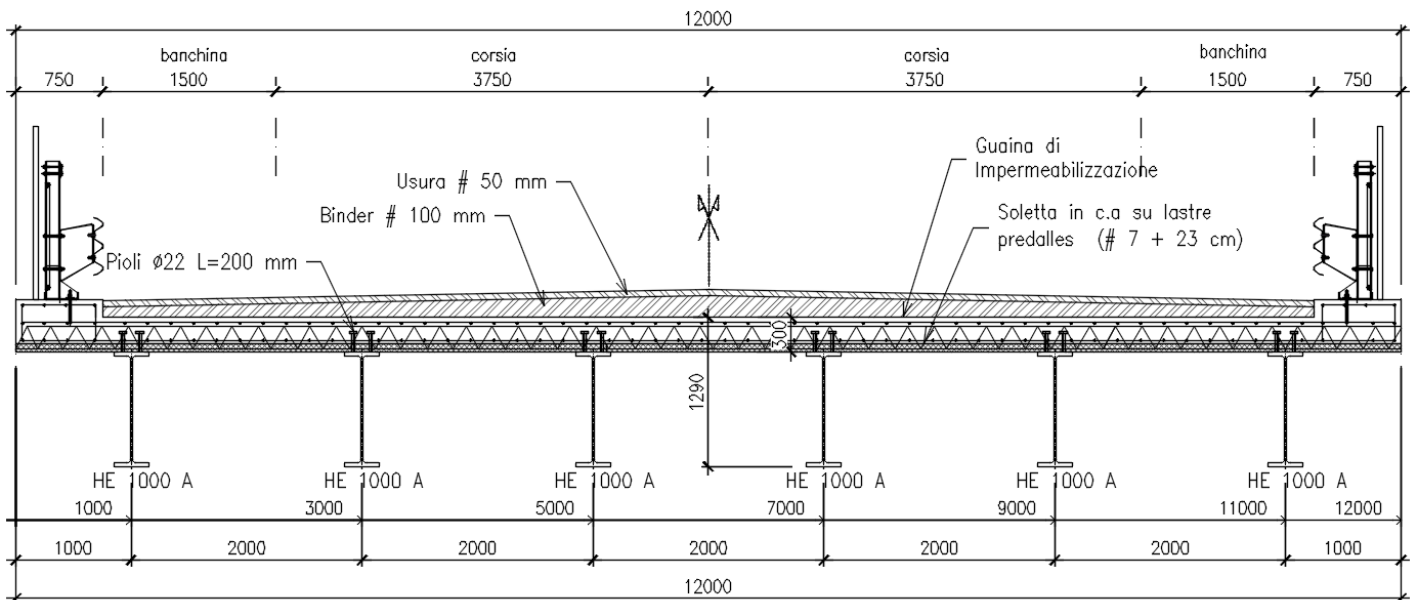
Figura 4.11 – Sezione tipo
