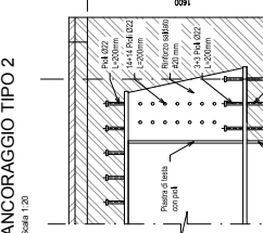
SISTEMI PER IL TRAVERSO IN CALCESTRUZZO SULLA PILA ANCORAGGIO TIPO 2 Scala 1/20
