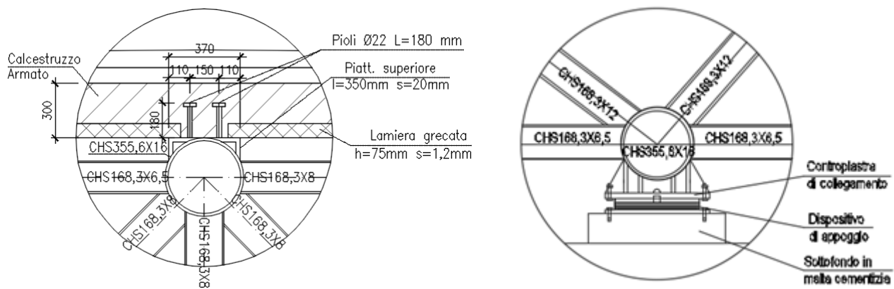
Figura 4.67 - Dettaglio soletta
