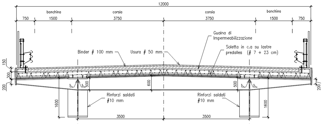
Figura 4.58 - Sezione tipo
