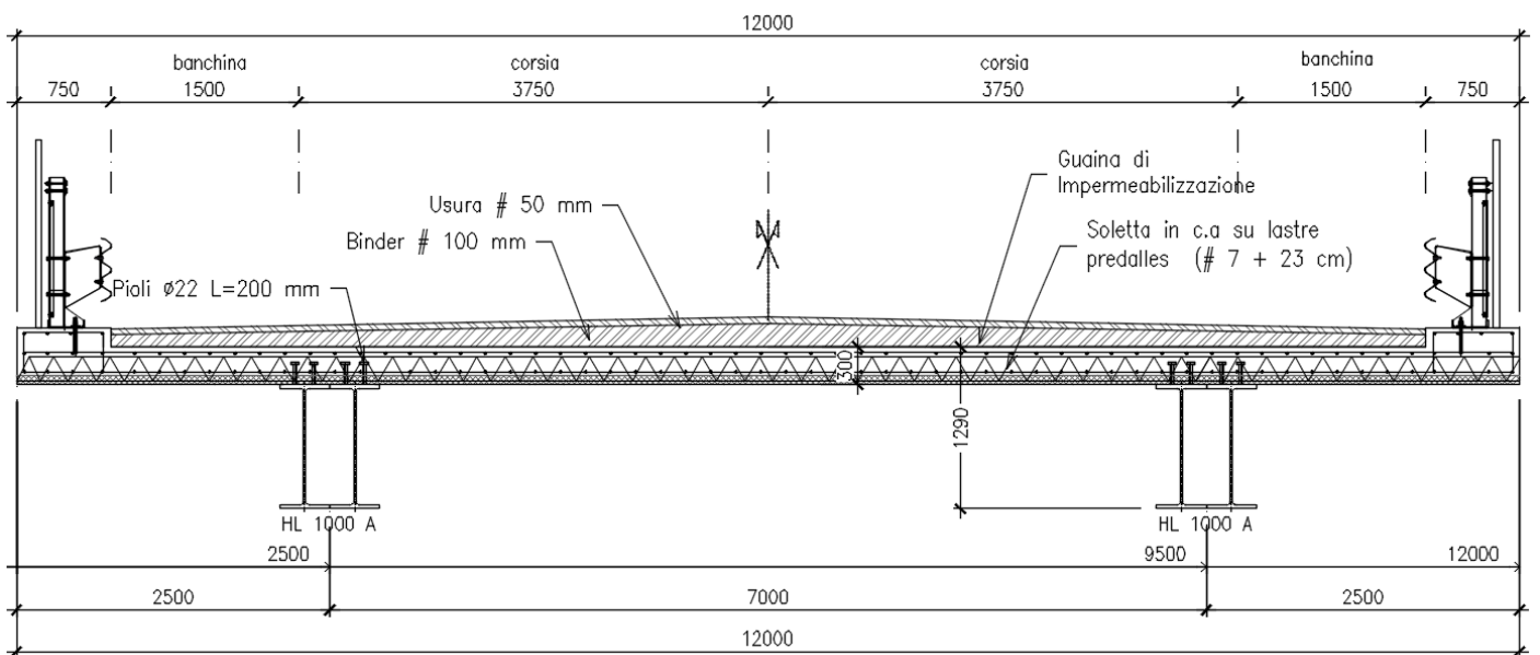
Figura 4.9 – Sezione tipo
