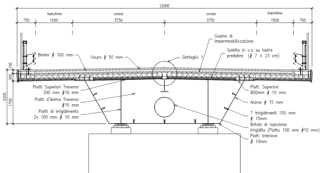
Figura 4.24 - Sezione tipo
