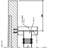
APPOGGIO IN CAMPATA Scala 1:20
