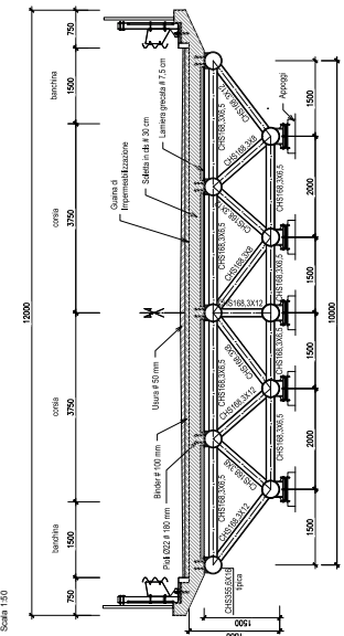
SEZIONE A-A Scala 1:50
