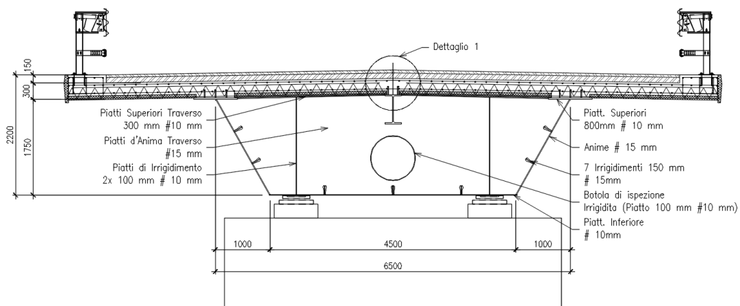
Figura 4.35 - Sezione all'appoggio
