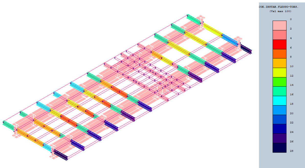
Figura 4.57 – Coefficiente di utilizzo flessio-torsionale soluzione tipo Travi a doppio T, bi-trave lamiera composta saldata
