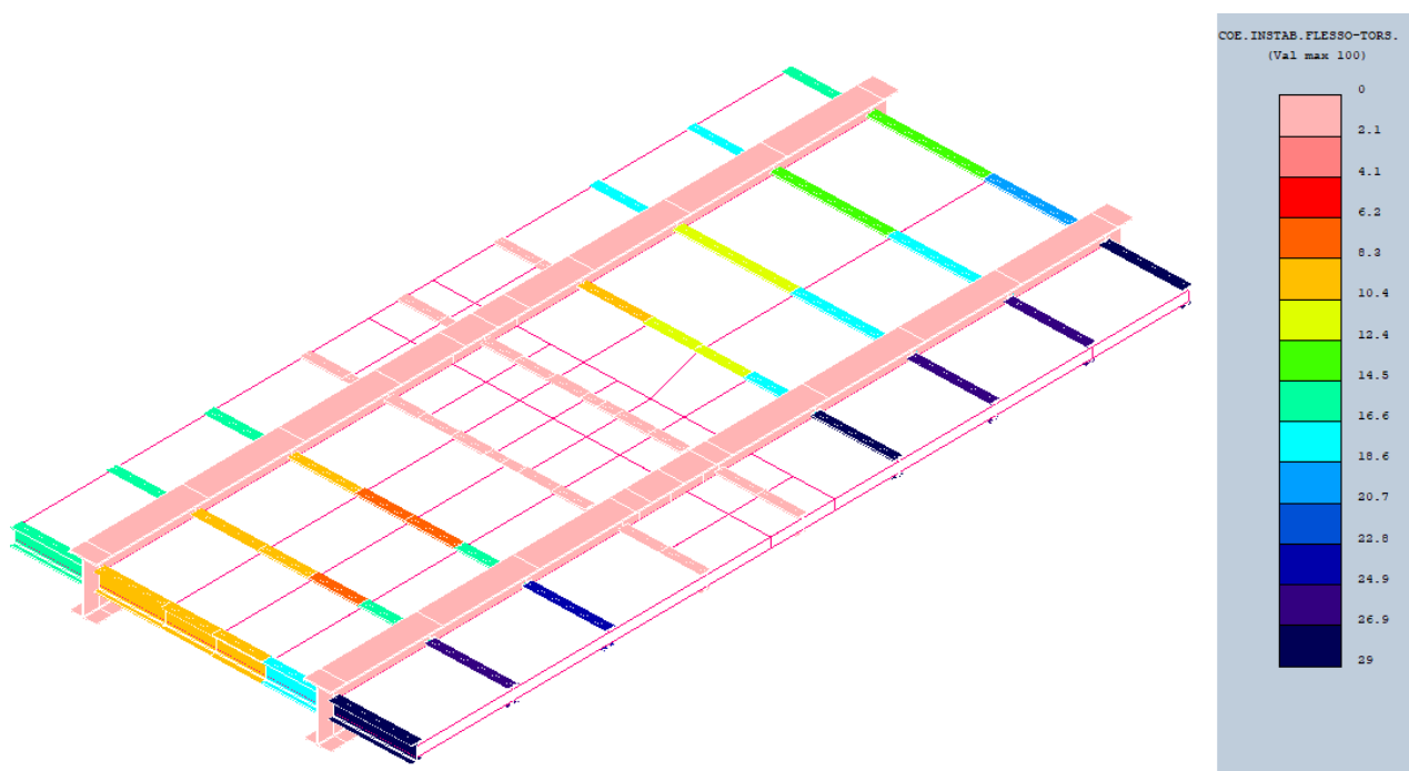
Figura 4.51 – Coefficiente di utilizzo flessio-torsionale soluzione tipo Travi a doppio T, bi-trave lamiera composta saldata
