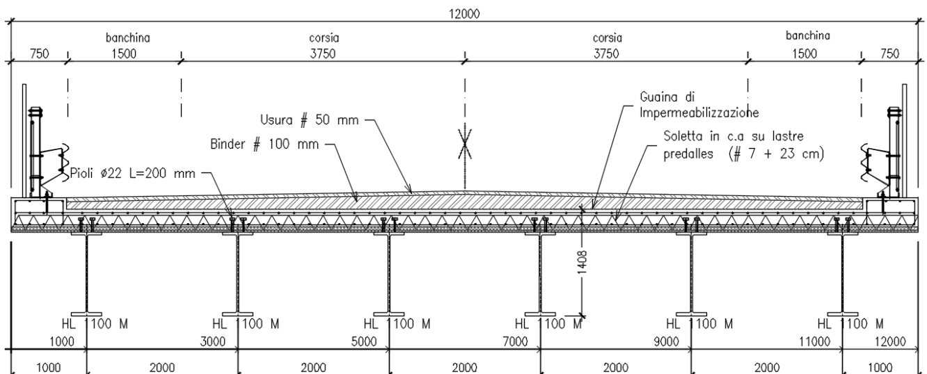
Figura 4.13 - Sezione tipo
