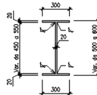
Figura 4.53 - Sezioni profili tipo
