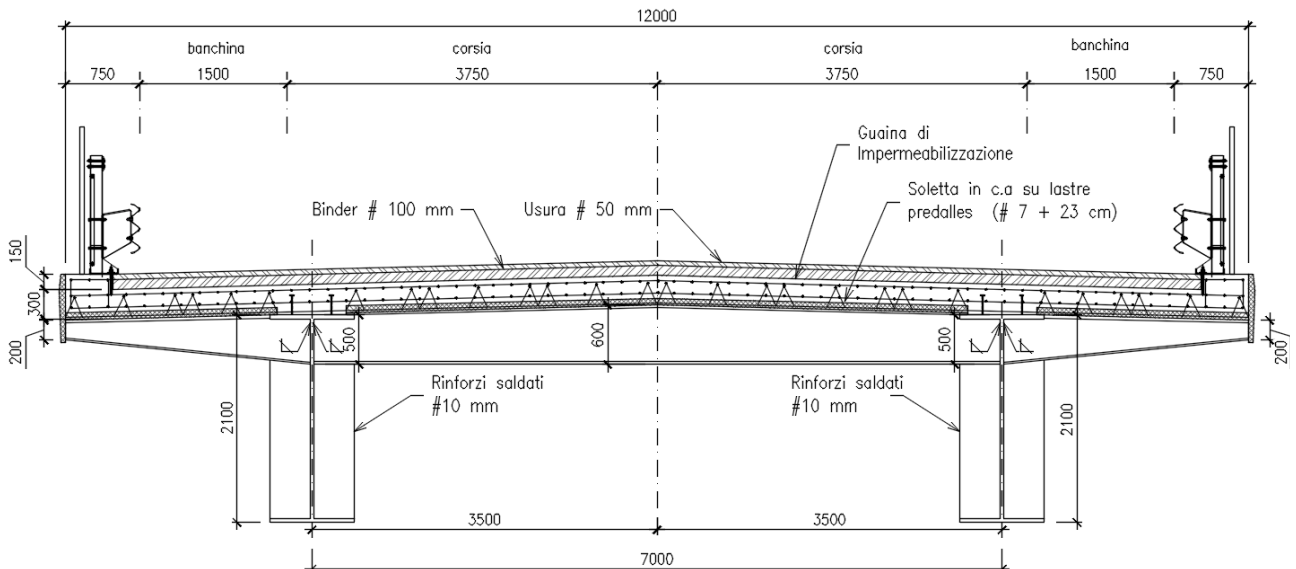
Figura 4.52 - Sezione tipo
