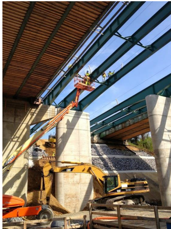
Figura 4.105 - Esempio di allargamento di ponte esistente con travi metalliche poggiate su nuovi appoggi
