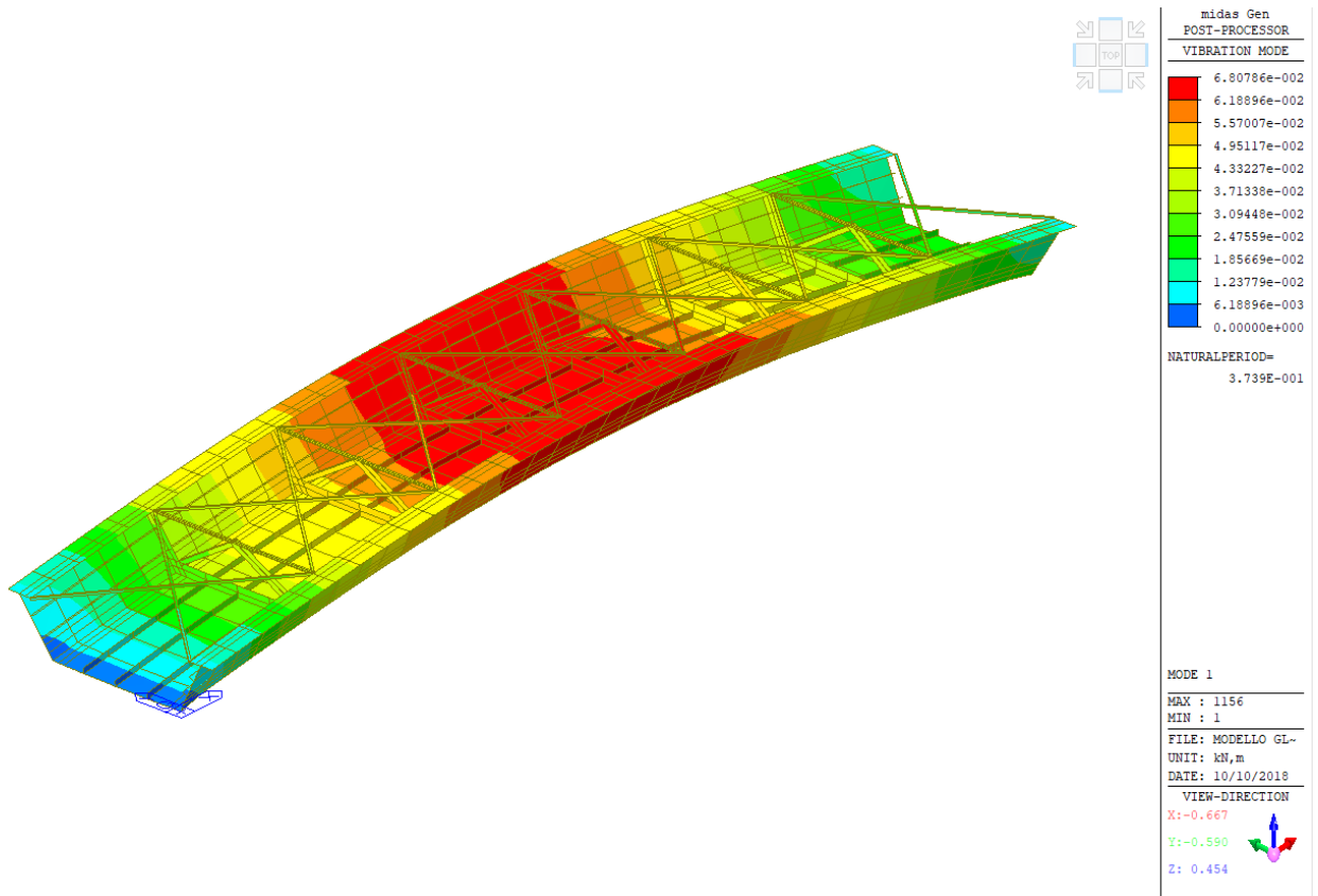
Figura 4.32 – Primo modo di vibrare verticale T=0.37 s
