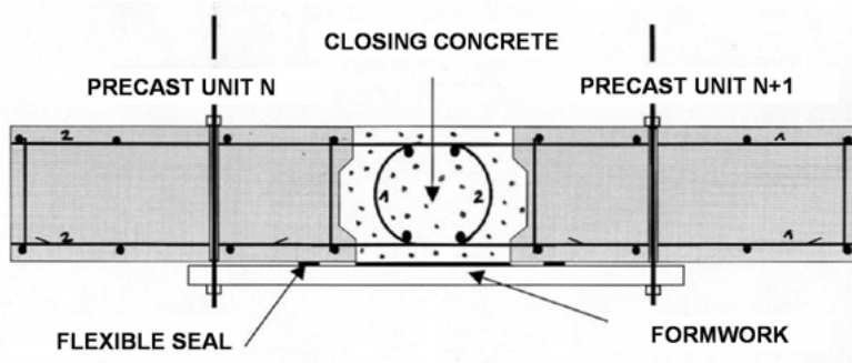
Figura 4.99 – Soluzione di getto con cassero tradizionale
