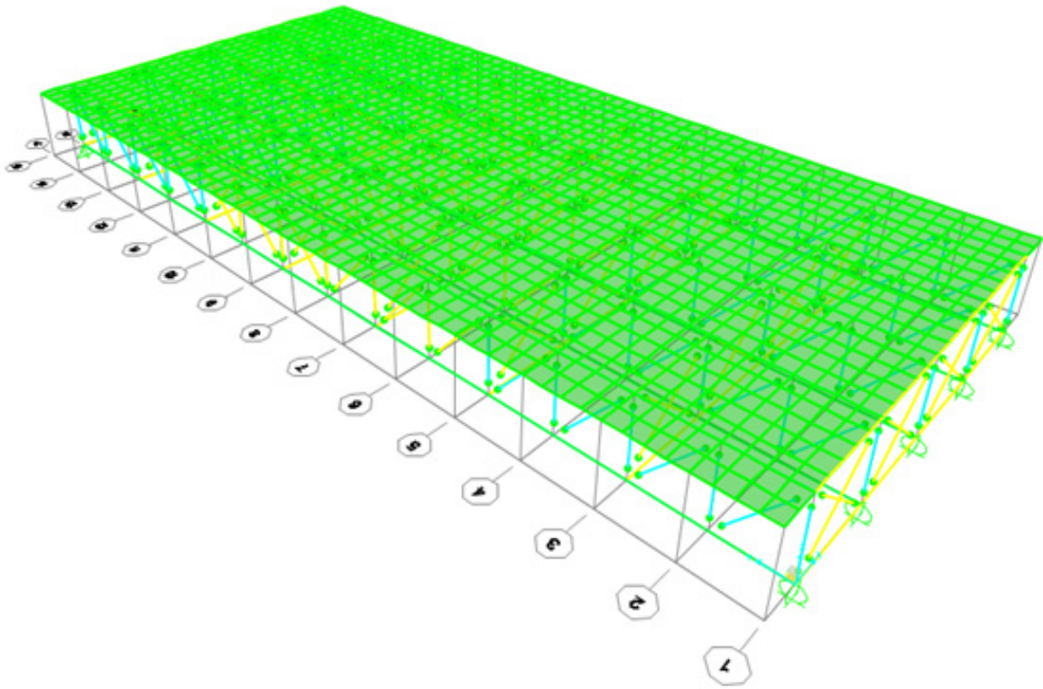
Figura 4.68 - Modello analitico
