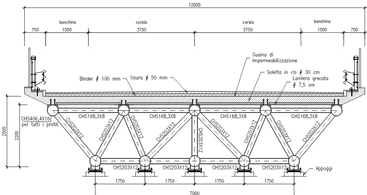
Figura 4.74 - Sezione tipo
