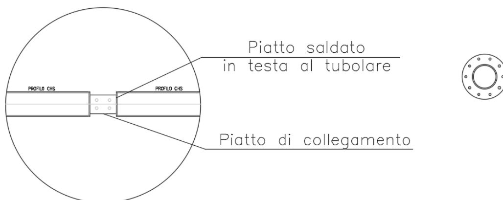
Figura 4.94 - Esempio nodo bullonato e sezione flangia
