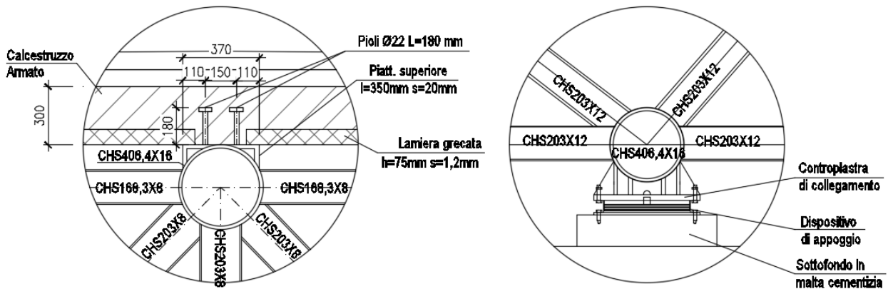
Figura 4.75 - Dettaglio soletta
