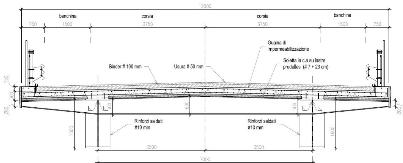
Figura 4.45 - Sezione tipo
