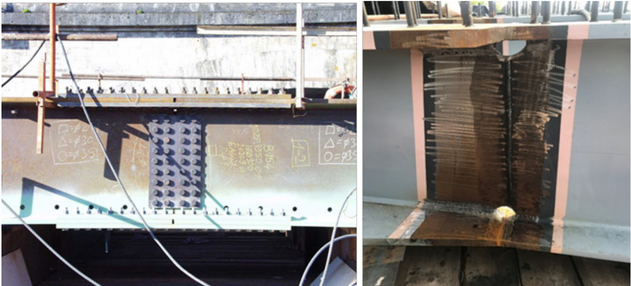
Figura 4.20 – Giunto bullonato e giunto saldato
