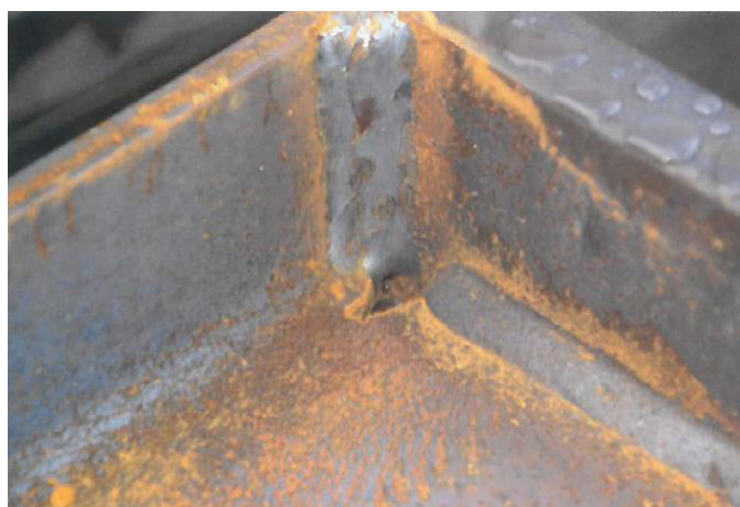
Figura 6.18 - La presenza del cordone di saldatura rende insufficiente la sezione del foro di drenaggio [35]
