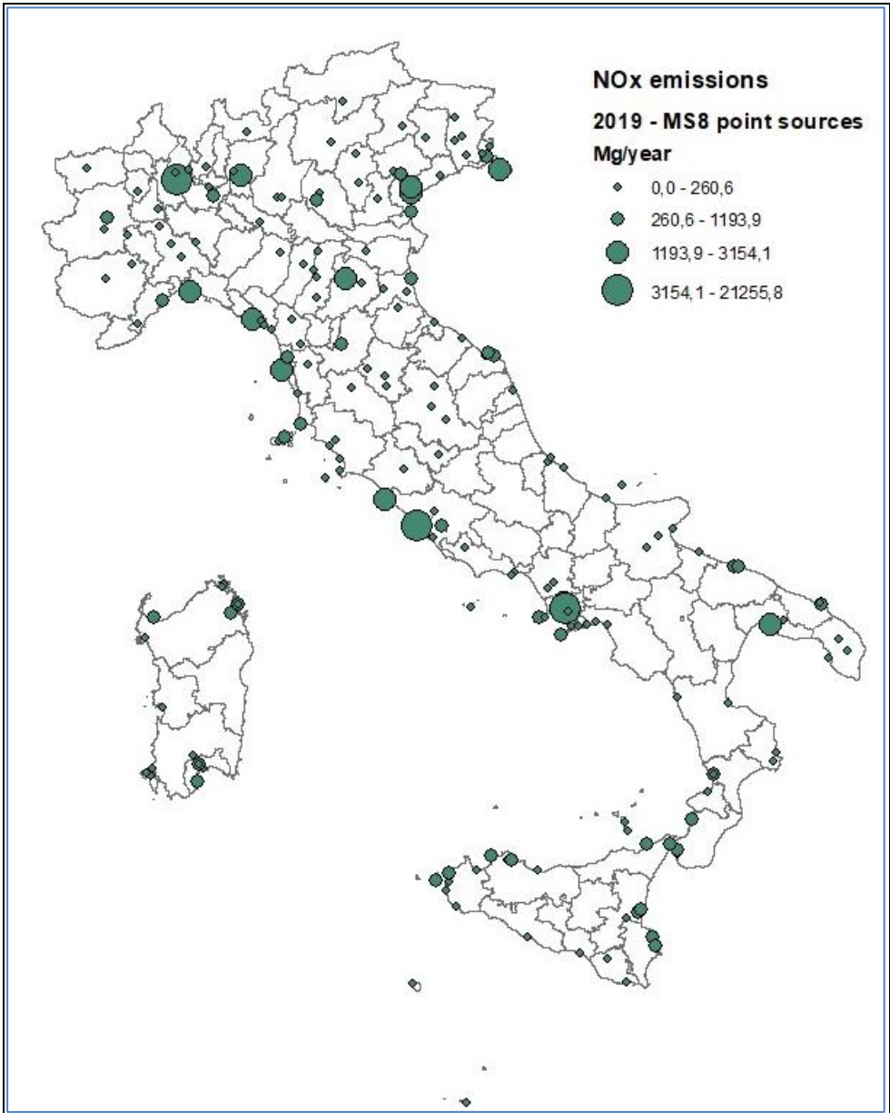
Figura 3.9.1 Emissioni di NOx (t) dal Macrosettore 08: Altre Sorgenti Mobili – Anno 2019
