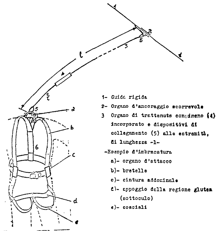
Figura 1 - Disegno schematico dell'attrezzatura - Nomenclatura
