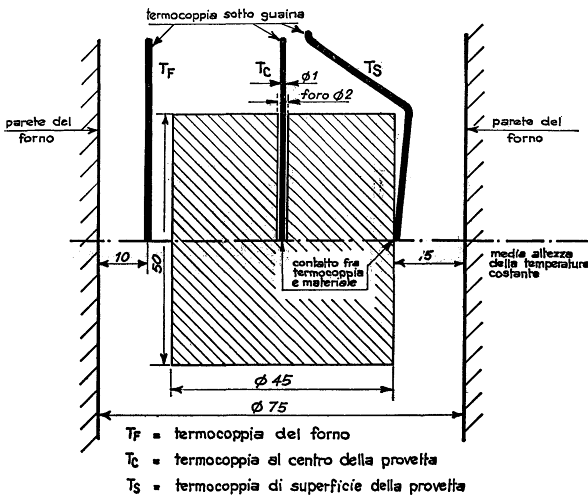
Fig. 2 — Posizione relativa del forno, della provetta e delle termocoppie
