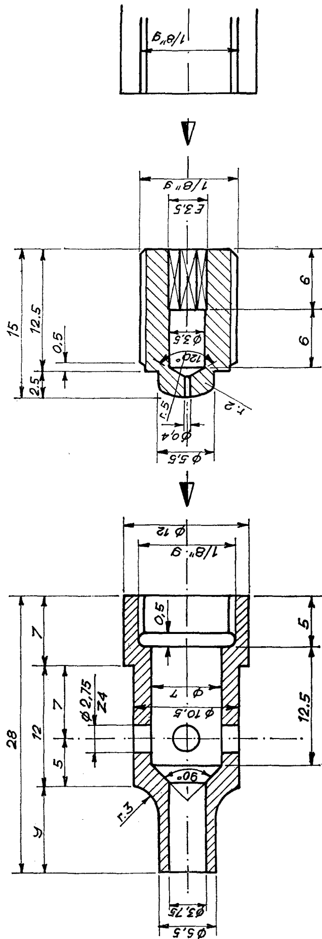
Fig. 5 — Bruciatore fiamma pilota ([materiale] ottone)
