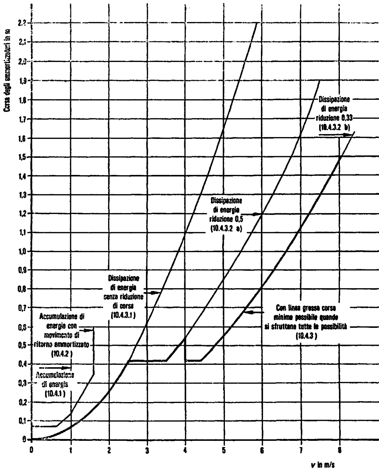
Fig. 3 — Grafico delle corse richieste per gli ammortizzatori (10.4)
