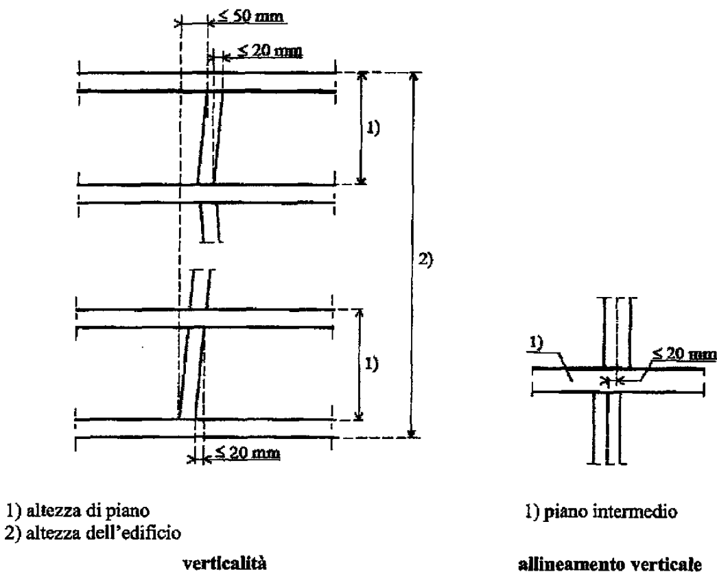
Fig. 3.1 - Massima deviazione della verticale
