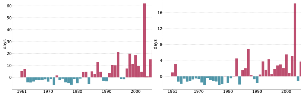
Figura 2.1: Serie delle anomalie medie annuali della frequenza (HWF), a sinistra, e della durata (HWD), a destra, delle onde di calore definite dall'EHF in Italia, rispetto alla media 1961-1990.
