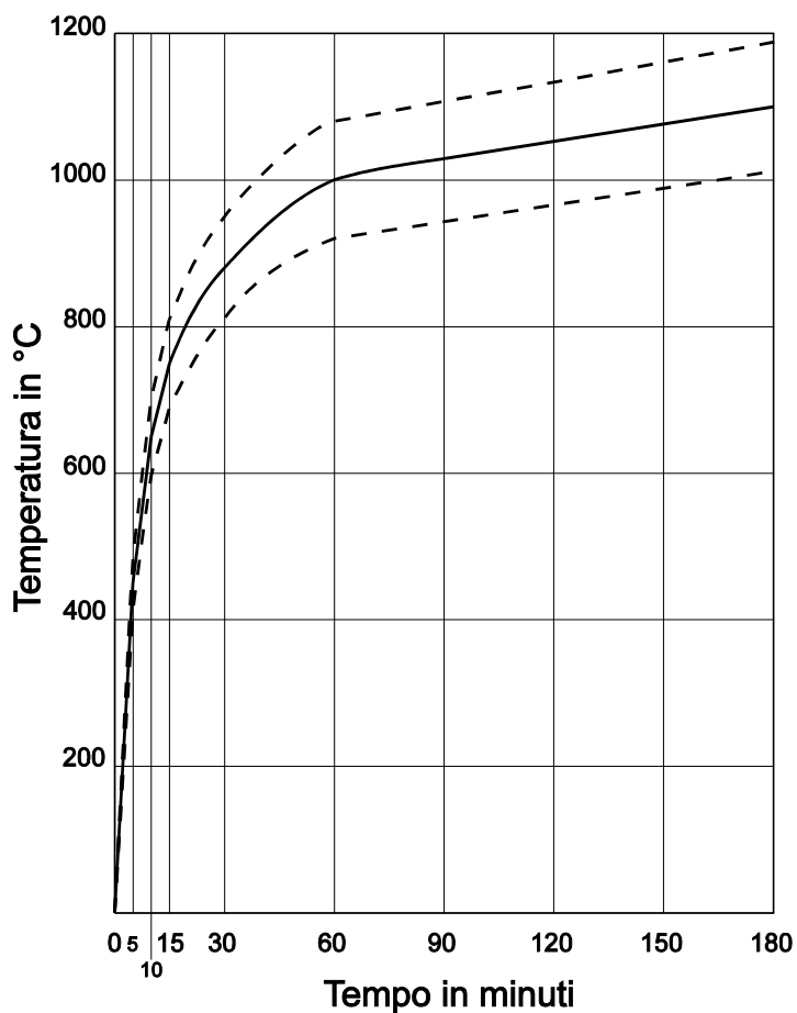
Fig. 2 - Curva temperatura-tempo
