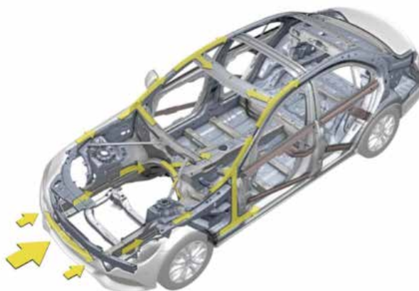
Distribuzione delle forze in un urto frontale
