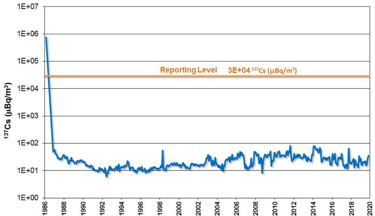
Figura 8.1 - Andamento della concentrazione di Cs-137 nel particolato atmosferico in Italia
