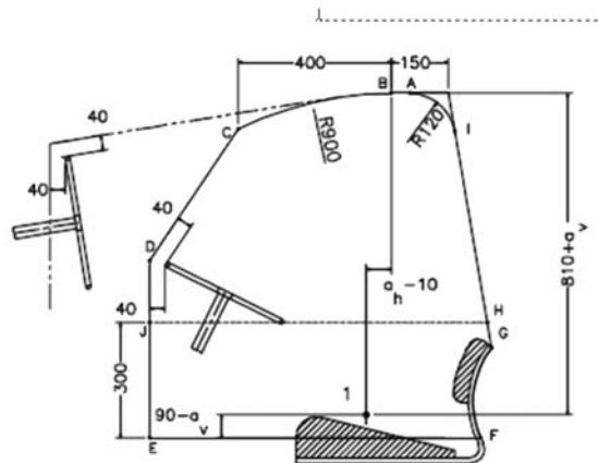
Figura 3.9.a Vista laterale Sezione nel piano di riferimento
