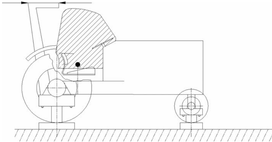
Figura 4.1.b Roll-bar posteriore
