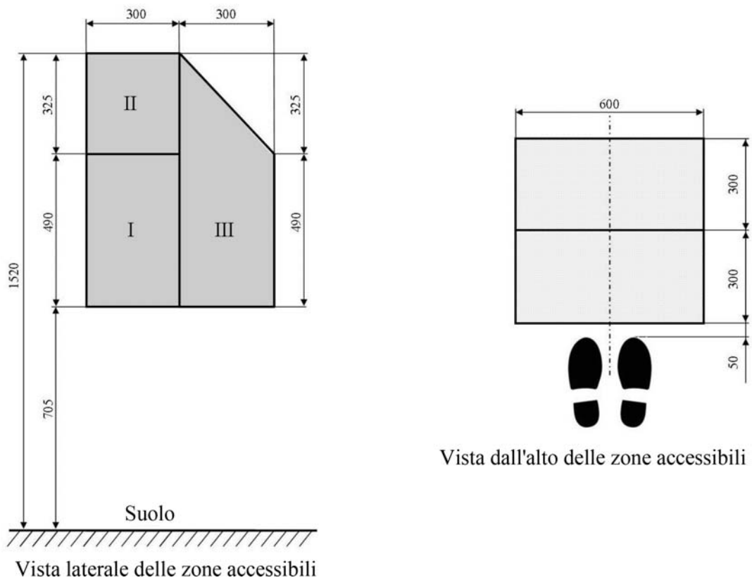
Figura 6.21 Zone accessibili (dimensioni in mm)
