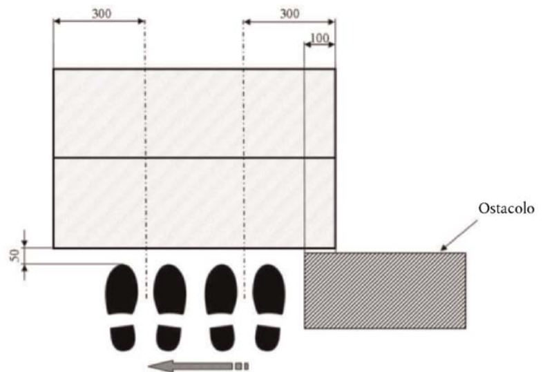
Figura 7.11 Spazio che racchiude le aree accessibili (Dimensioni in mm)
