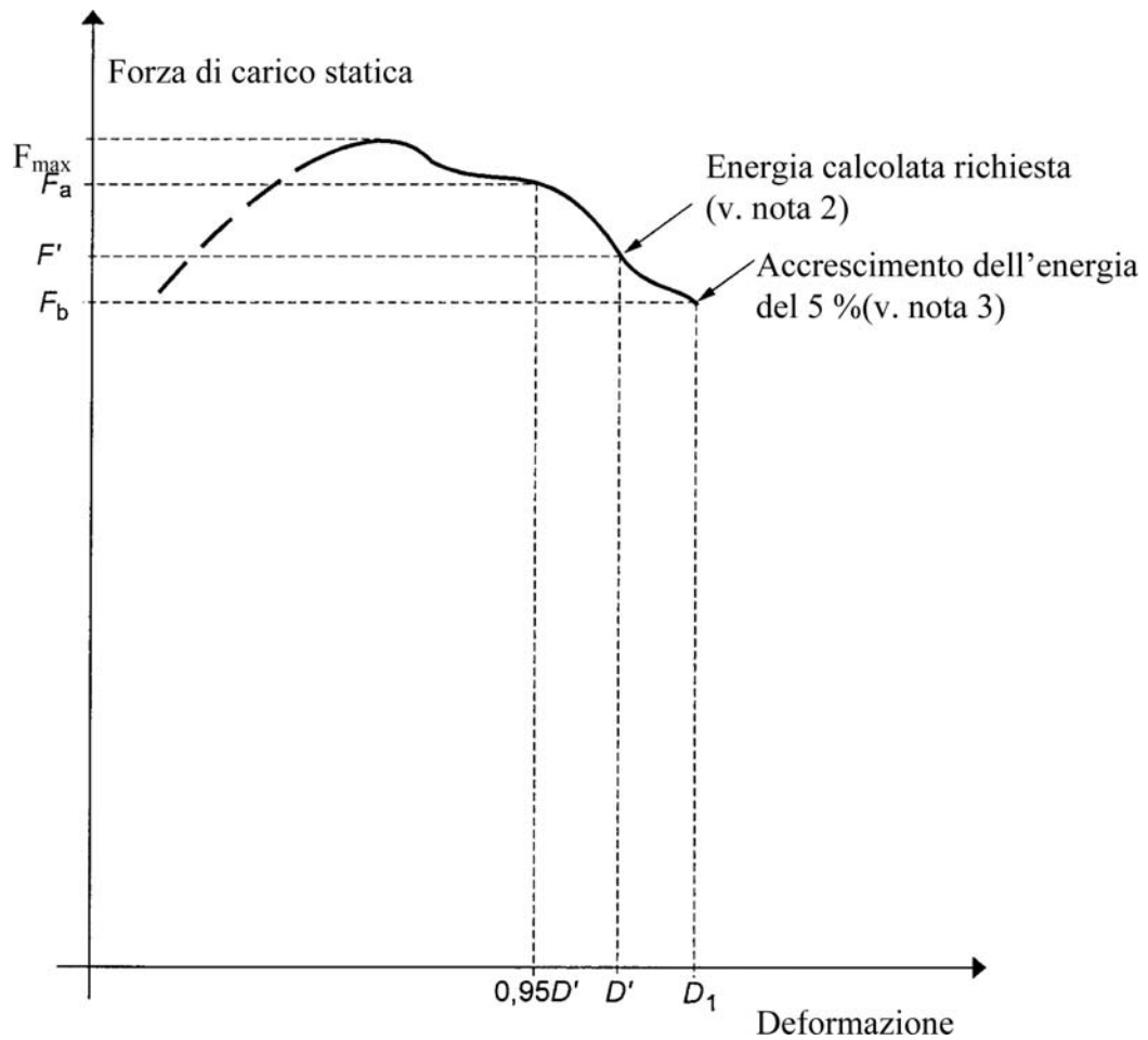
Figura 7.6 Curva forza/deformazione Prova di sovraccarico necessaria
