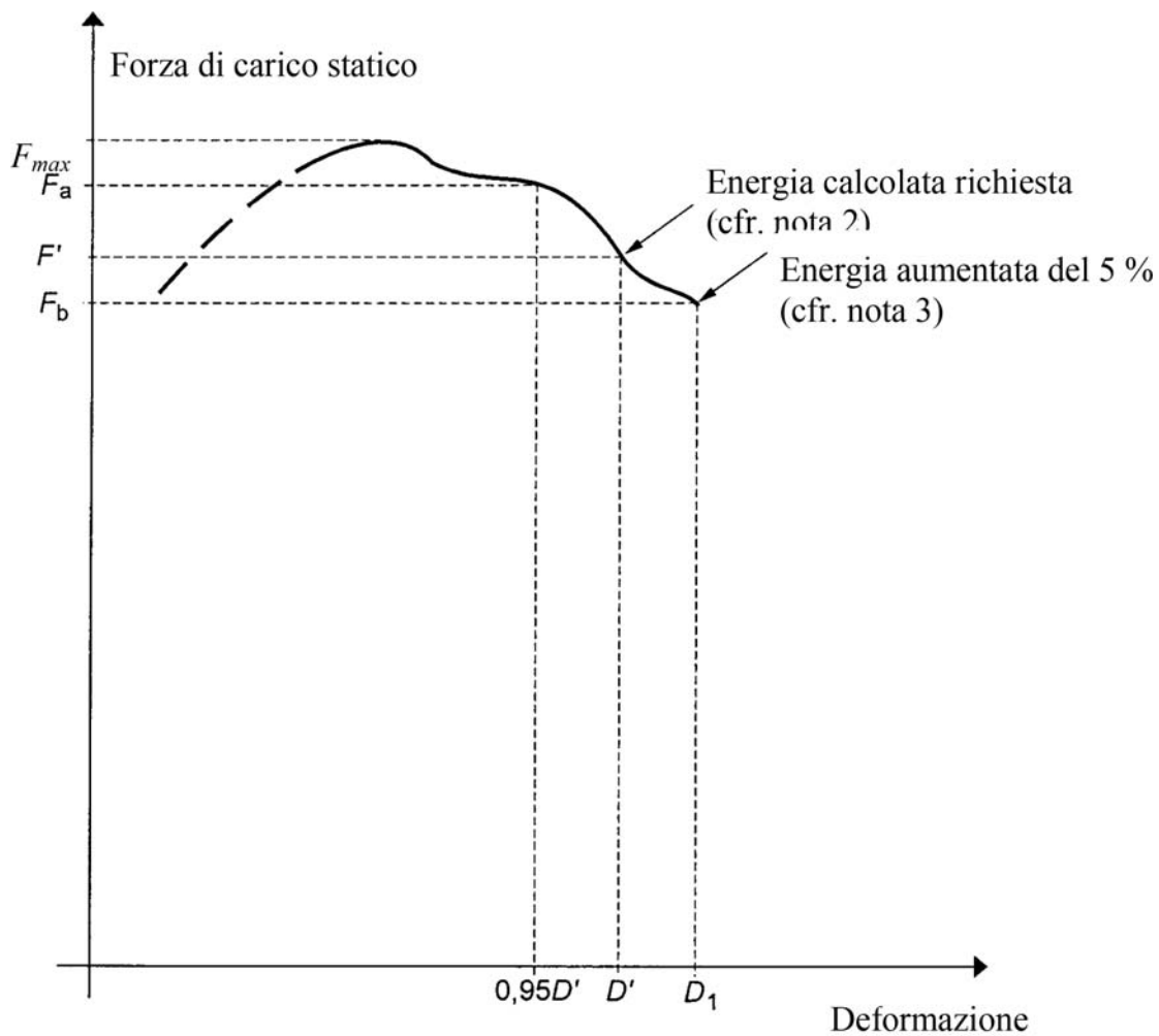
Figura 4.15 Curva forza/deformazione Prova di sovraccarico necessaria
