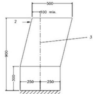
Figura 3.9.b Vista posteriore o anteriore
