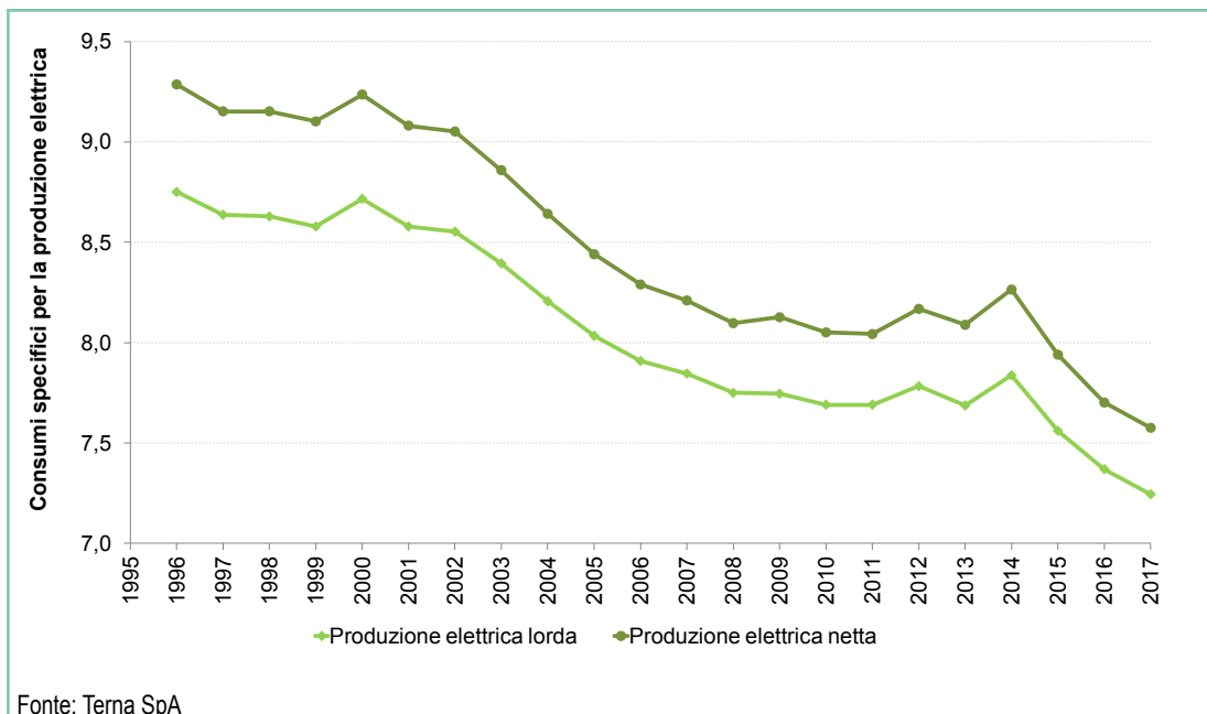
Figura 3.7: Consumi specifici medi di combustibile della produzione lorda e netta di energia elettrica da fonti fossili
