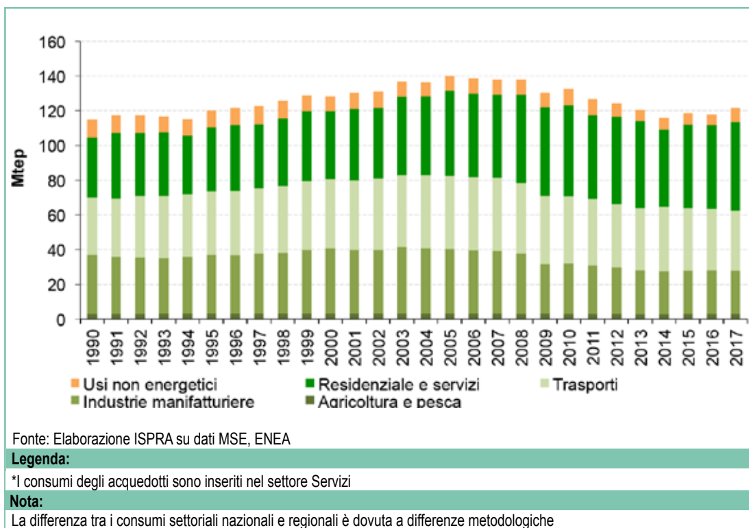
Figura 3.5: Consumi finali di energia per settore economico
