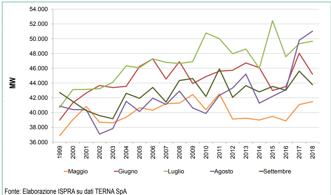
Figura 3.17: Punta oraria di fabbisogno energetico nei mesi estivi
