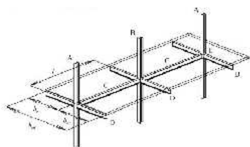
Fig. 7.6.2 - Definizione degli elementi in una struttura intelaiata
