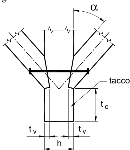
Figura 8-1 - Unione a dente simmetrico
