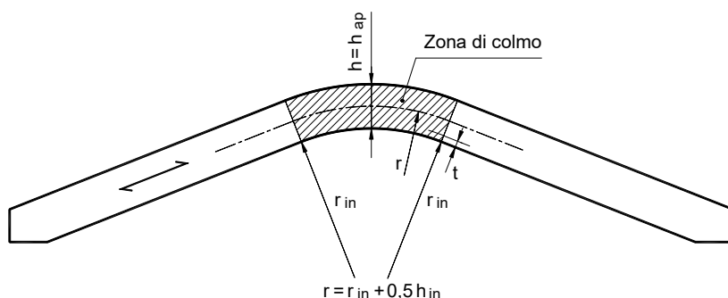
Figura 7-7 – Trave curva
