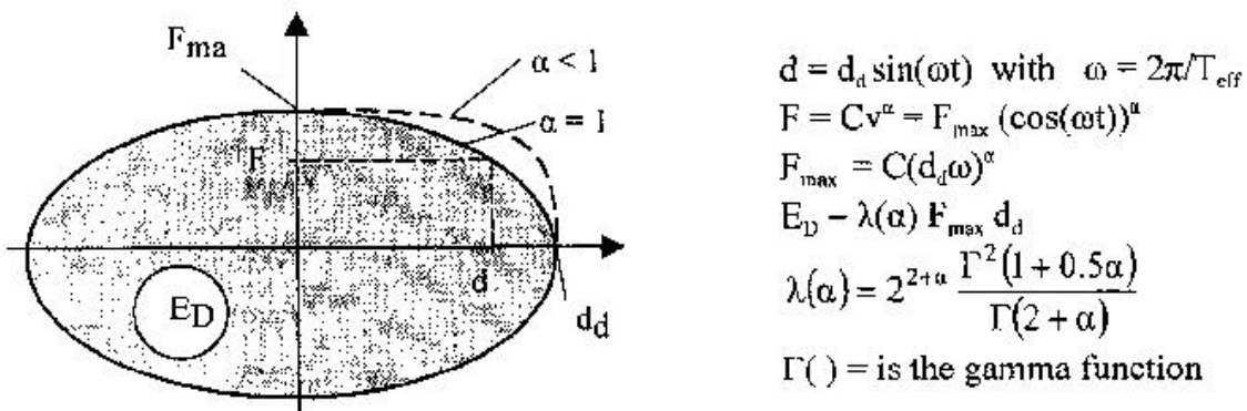
Figura 10.2 – Dispositivi a comportamento viscoso
