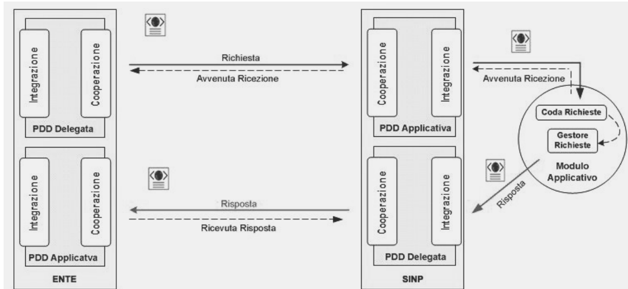
Figura 2 - Profilo Asincrono
